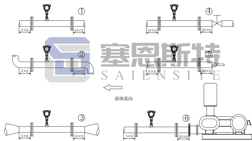
安装前后直管段图
