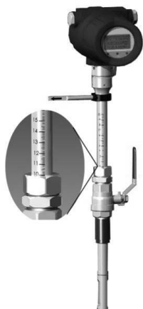
图 1 适用管径 DN65 以上 DN2000 以下 精简型热式气体质量流量计
