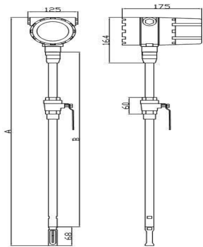
精简型插入型外形尺寸 单位：mm
